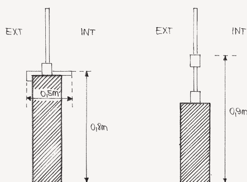
Figure 17 : hauteurs allèges
